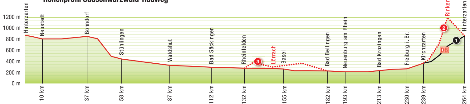
Höhenprofil Südschwarzwald-Radweg
